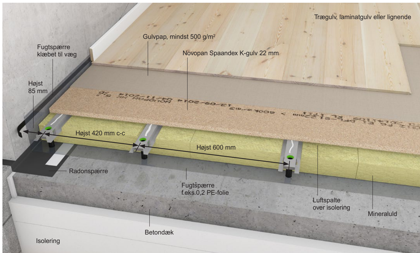
Figur 1 Novopan Spaandex K-gulv 22 mm på stålstrøer – system Granab 3000N. Strølaget udføres med randstrøer langs alle vægge og en strø-afstand i afstanden i første fag langs væg på 420 mm c-c.
